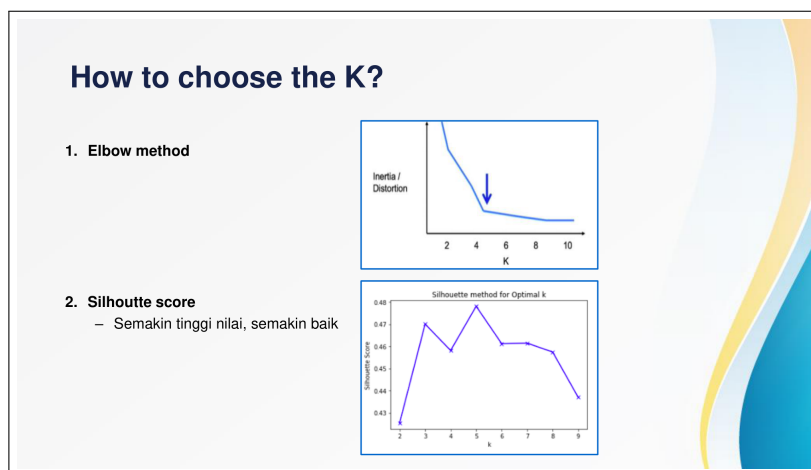
Gambar 8: Penentuan jumlah klaster optimal memakai kurva Elbow dan Silhouette Score [11].
